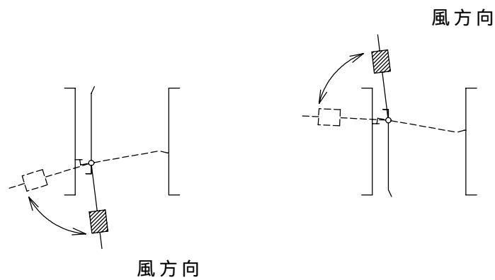
垂直取付の場合のバランスウエイトの取付角度
